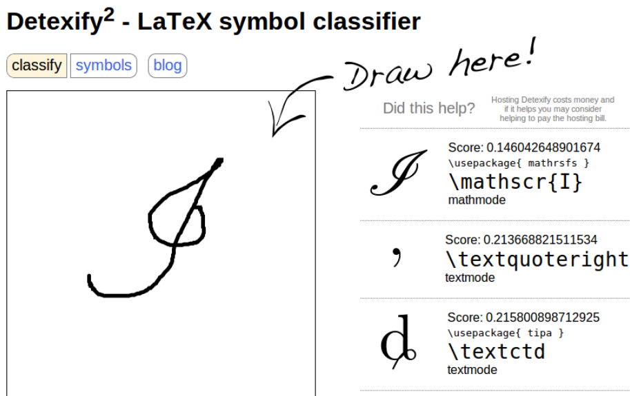
Figura 1.5. Detexify
